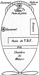
Plan schématique de la nacelle avant.
